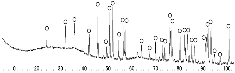
Itokawa RA-QD02-0028 O:olivine
